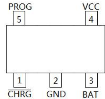
SOT23-5L
