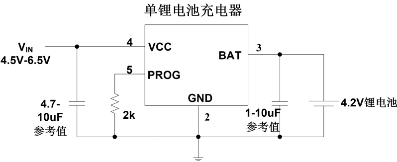
基本电路
