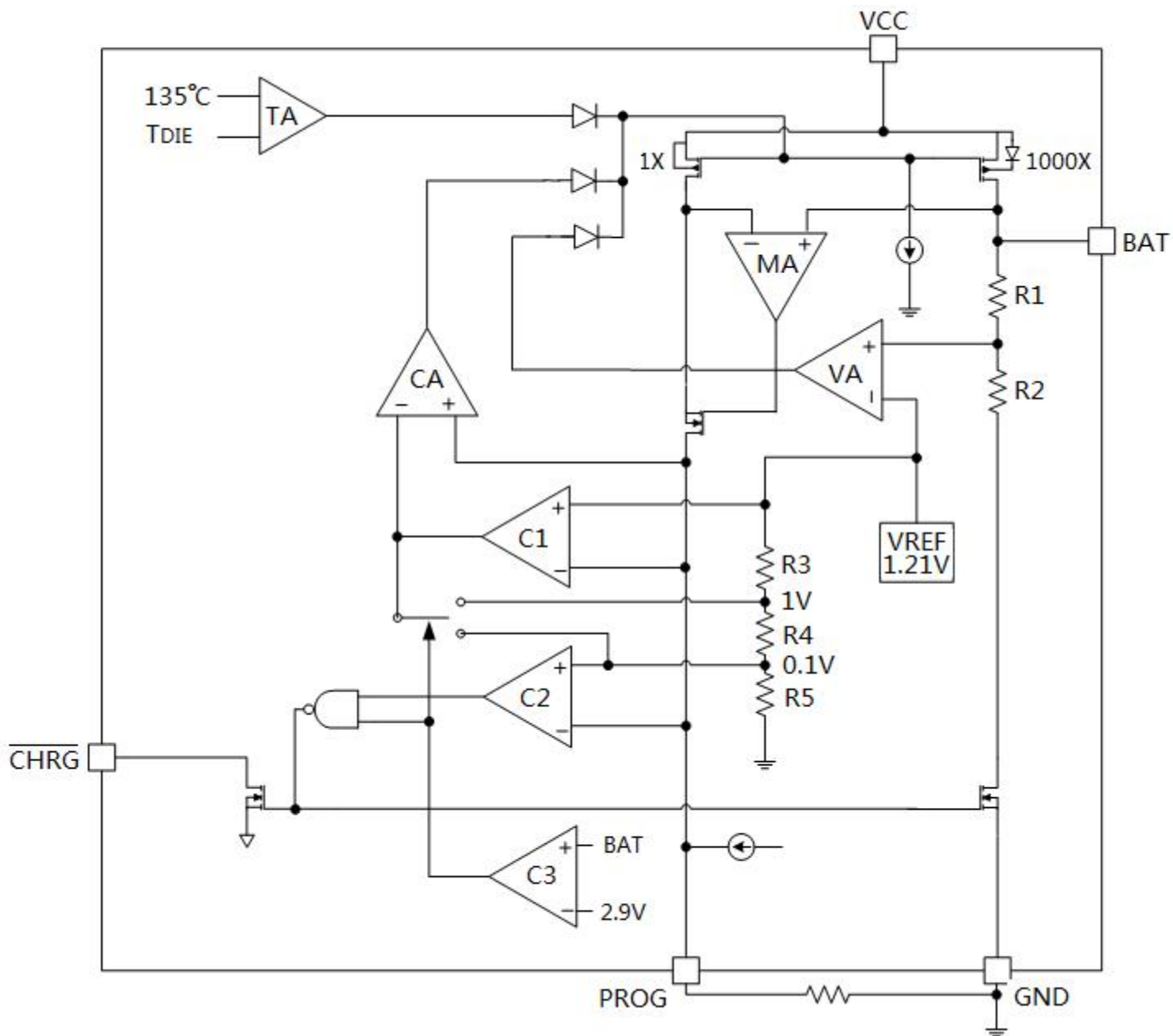
结构框图
