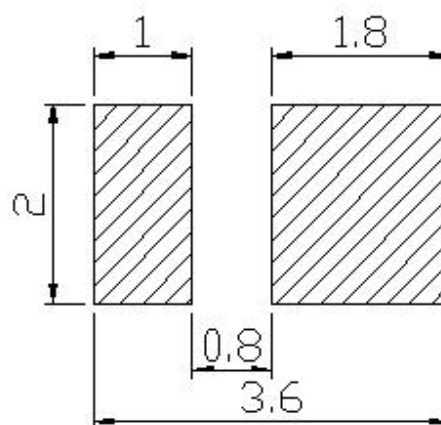
焊盘建议图
