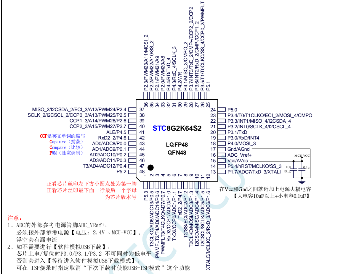
STC8G2K64S2-36I-LQFP48/QFN48 最小系统 示意图
