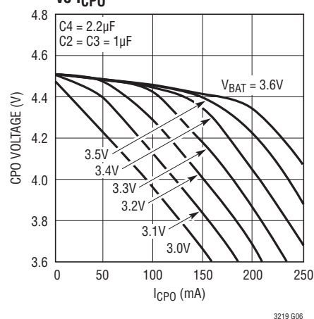
1.5x Mode CPO Voltage vs I_{\text{CPO}}
