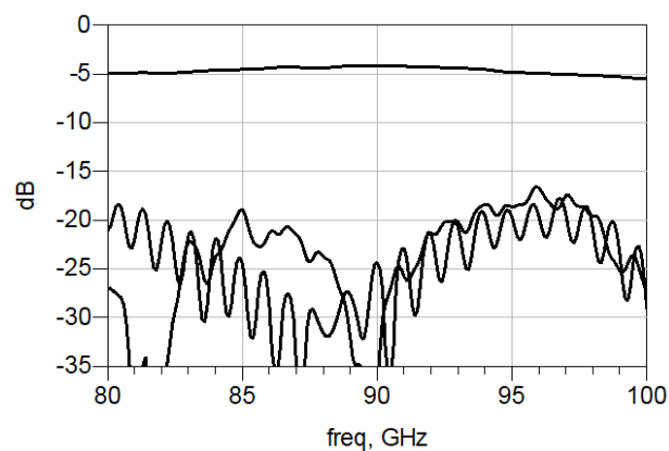
Thru S-Parameters
