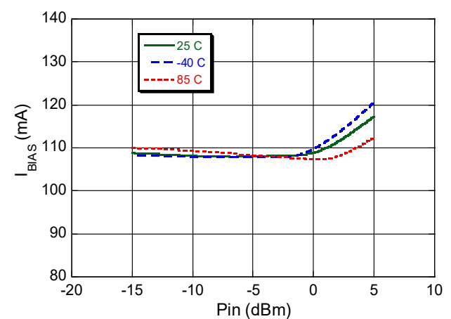
I_{BIAS} @ 15 GHz
