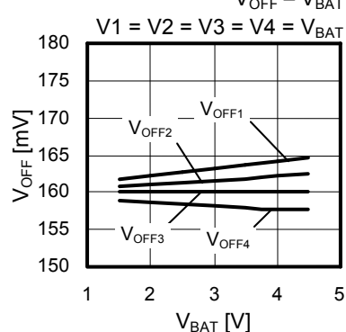
S-8243BAF V_{OFF} - V_{BAT}
