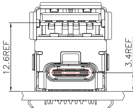
HIGE RISE USB3.1+USB TYPE C
