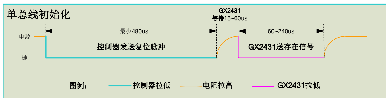
图 9. 初始化时序
