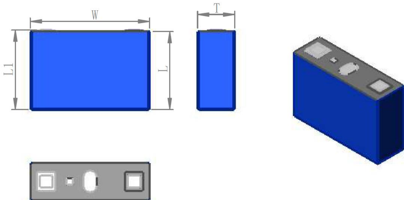
电芯尺寸Cell dimension
