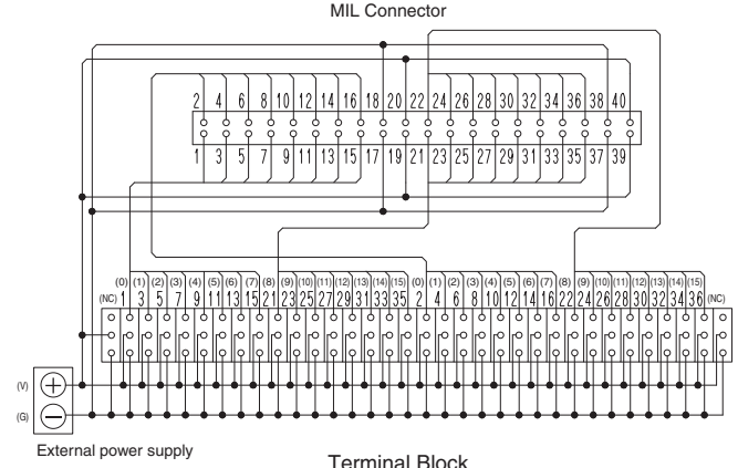
XW2R-P32GD-C3-COM
