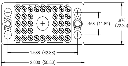
36 PIN RECEPTACLE
