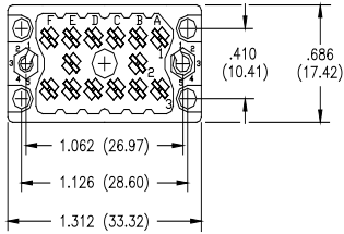
36 PIN RECEPTACLE
