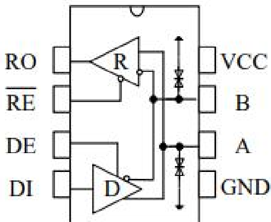
图 1 ESM3085E 引脚分布图
