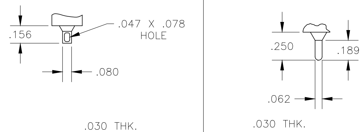
Z WIRE LUG Z3 QUICK CONNECT
