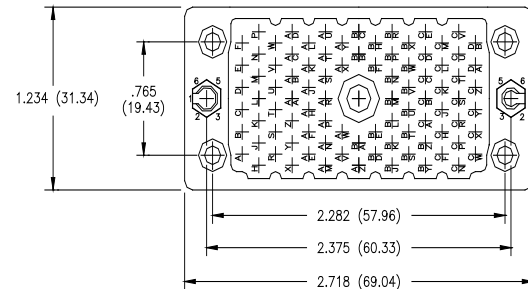
120 PIN RECEPTACLE
