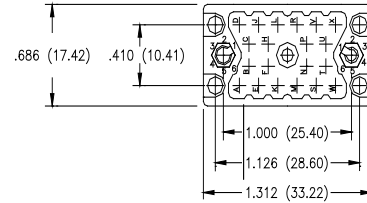
20 PIN RECEPTACLE
