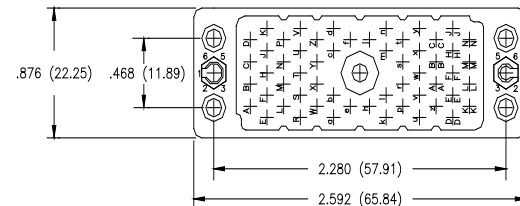
90 PIN RECEPTACLE
