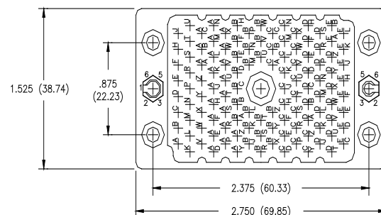
120 PIN RECEPTACLE
