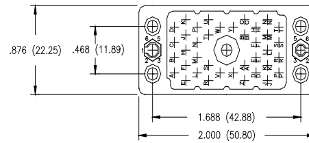
56 PIN RECEPTACLE
