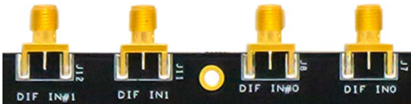
Figure 5. CLKIN0/CLKIN1 Inputs
