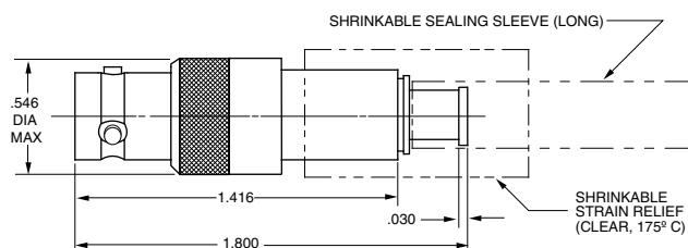
CJ70C-202 Shown
