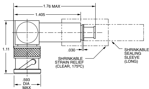
PLR74C-201 Shown
