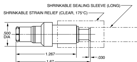
PL73C-202 Shown
