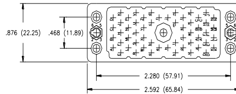
90 PIN RECEPTACLE
