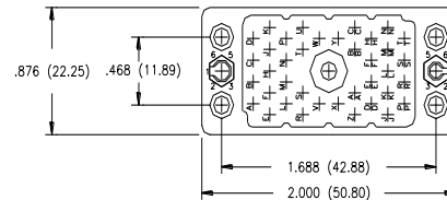
56 PIN RECEPTACLE
