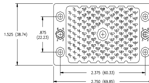
120 PIN RECEPTACLE
