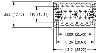
20 PIN RECEPTACLE
