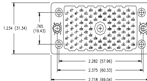
120 PIN RECEPTACLE
