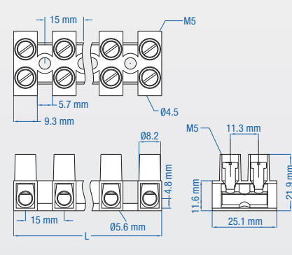
HE16 DIMENSIONS
