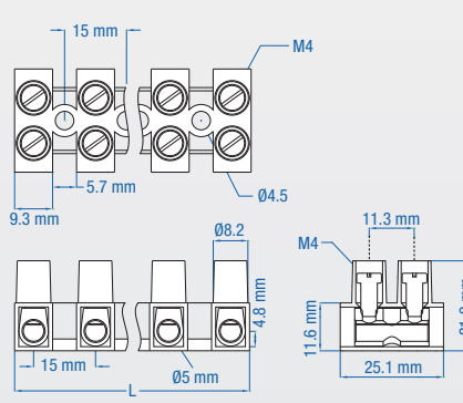
HE10 DIMENSIONS
