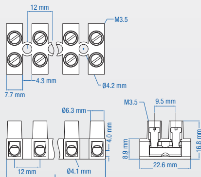
HE6 DIMENSIONS
