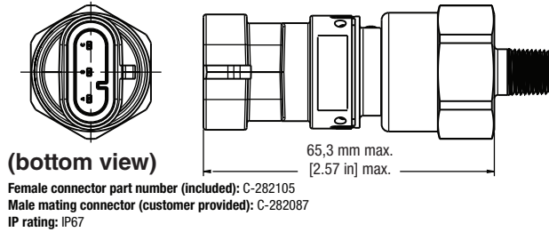
Figure 15. Deutsch 3-pin
