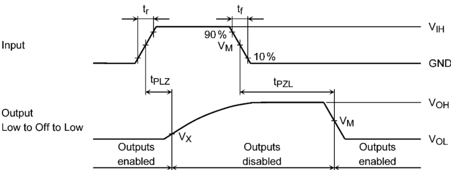
Fig. 9.8.1 t_{PLZ} , t_{PZL}
