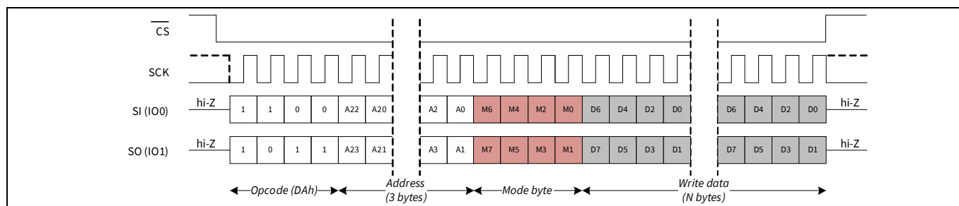
Figure 44 DPI 模式下的快速写入 (FAST_WRITE)
