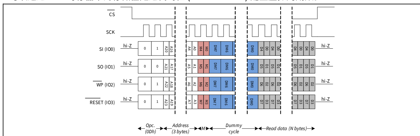
Figure 58 QPI 模式下的 DDRFR
