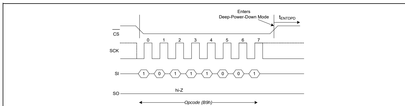
Figure 99 SPI 模式下的 DPD 进入
