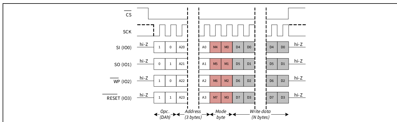
Figure 45 QPI 模式下的快速写入 (FAST_WRITE)
