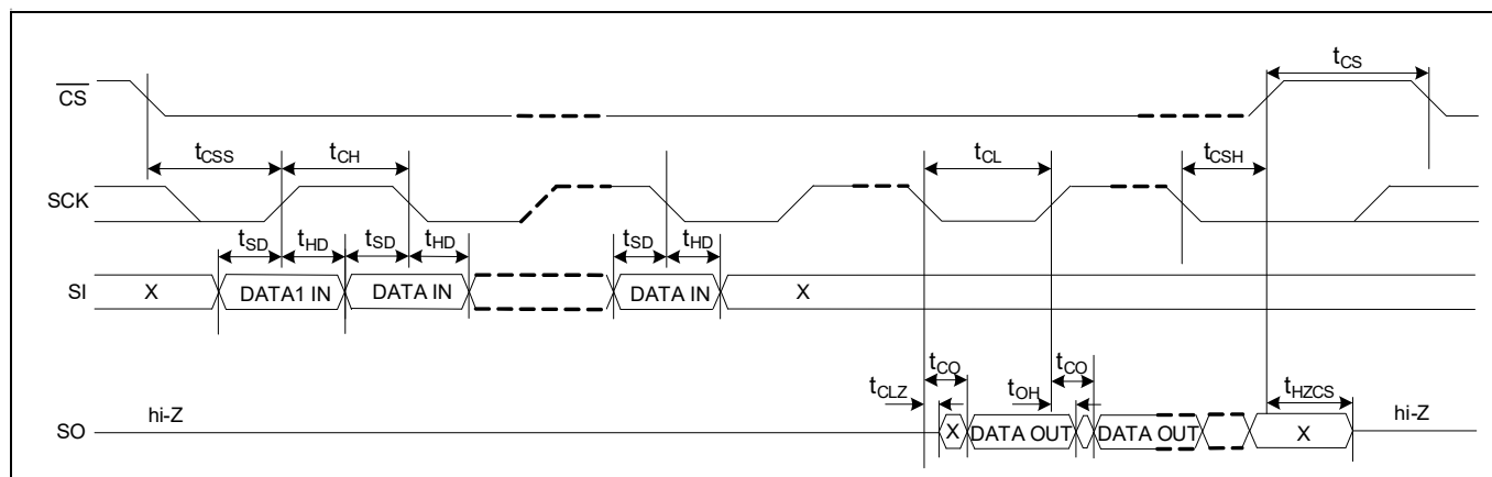
Figure 117 SPI 切换时序 — 单线 IO, DDR
