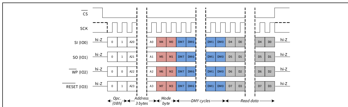
Figure 57 QPI 模式下的 FAST_READ 指令
