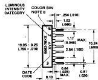
A,B SIDE
