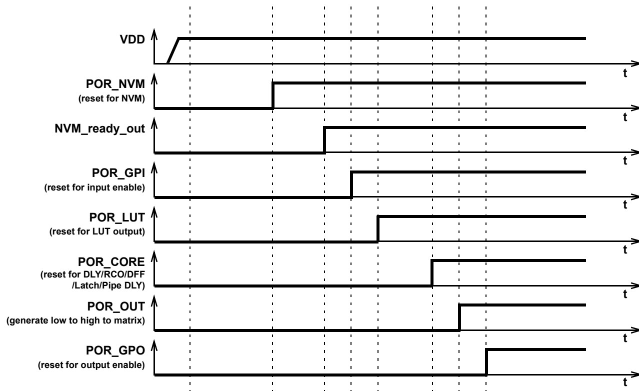
Figure 122. POR sequence
