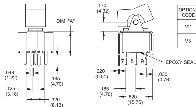
3PDT
