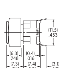
Extended Actuator
