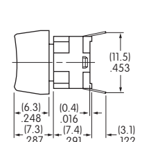
Extended Actuator
