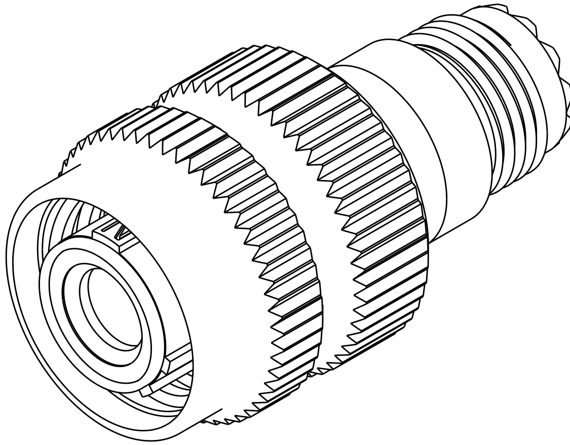
SCALE 4:1
