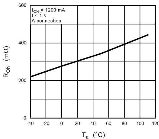
Fig. 13.5 R_{ON} - T_a
