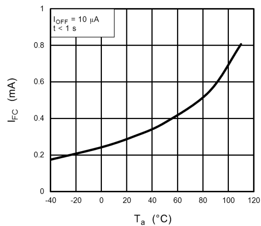
Fig. 13.6 I_{FC} - T_a
