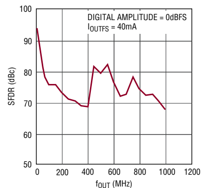
SFDR vs f_{OUT} , f_{DAC} = 2.5\text{Gps}
