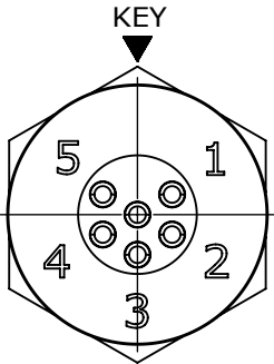
WIRING END W7282-6SG-P-300 SHOWN
