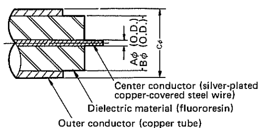
Semi-rigid cables
