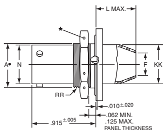
LJT07RP (MS27468P)
