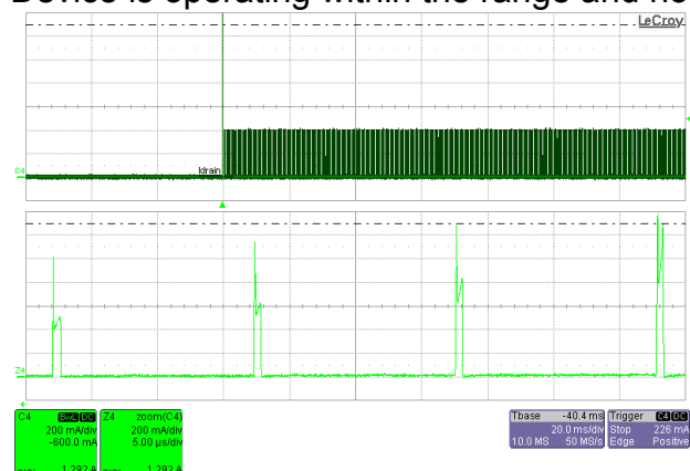
Figure 24 – LYT0006P Output Short. Ch4: I_{DRAIN} ; 0.2 A / div. Time Scale: 20 ms / div. Z4: V_{DS} ; 0.2 A / div. Zoom Time Scale: 5 \mu s / div.
