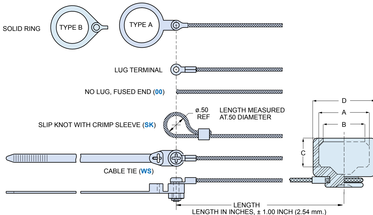
780-001 AND 780-002 DIMENSIONS
