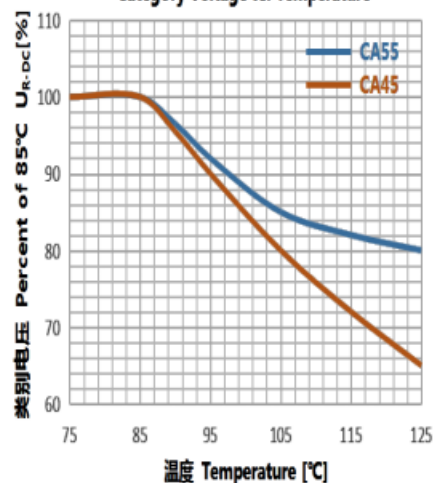
类别电压与温度的关系 Category Voltage vs. Temperature
