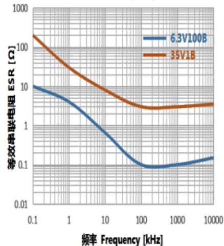
等效串联电阻与频率的关系 ESR vs. Frequency
