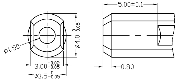
轴心部尺寸详图
