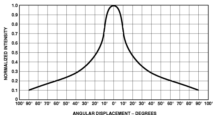
Figure 9. HLMP-Q102/-Q152
