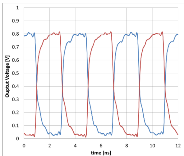
Figure 24. 250MHz HCSSL
