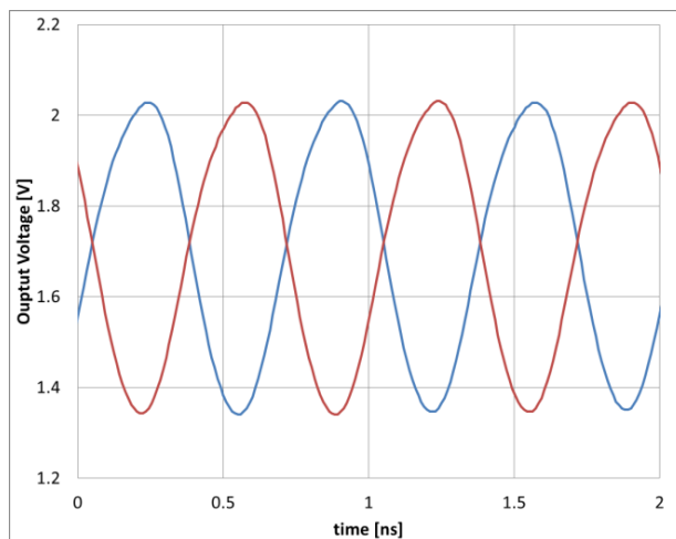
Figure 20. 1.5GHz LVPECL
