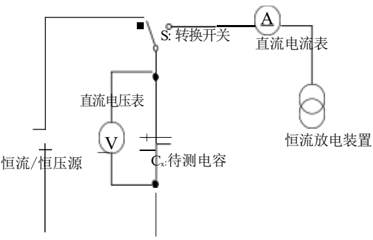
图 1. 容量测试电路
