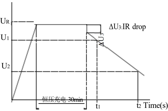
图 2. 充放电曲线图
