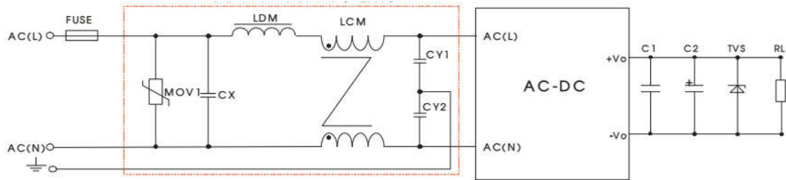
图 2 EMC 解决方案推荐电路
