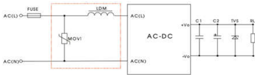
图 1 一般应用推荐电路
