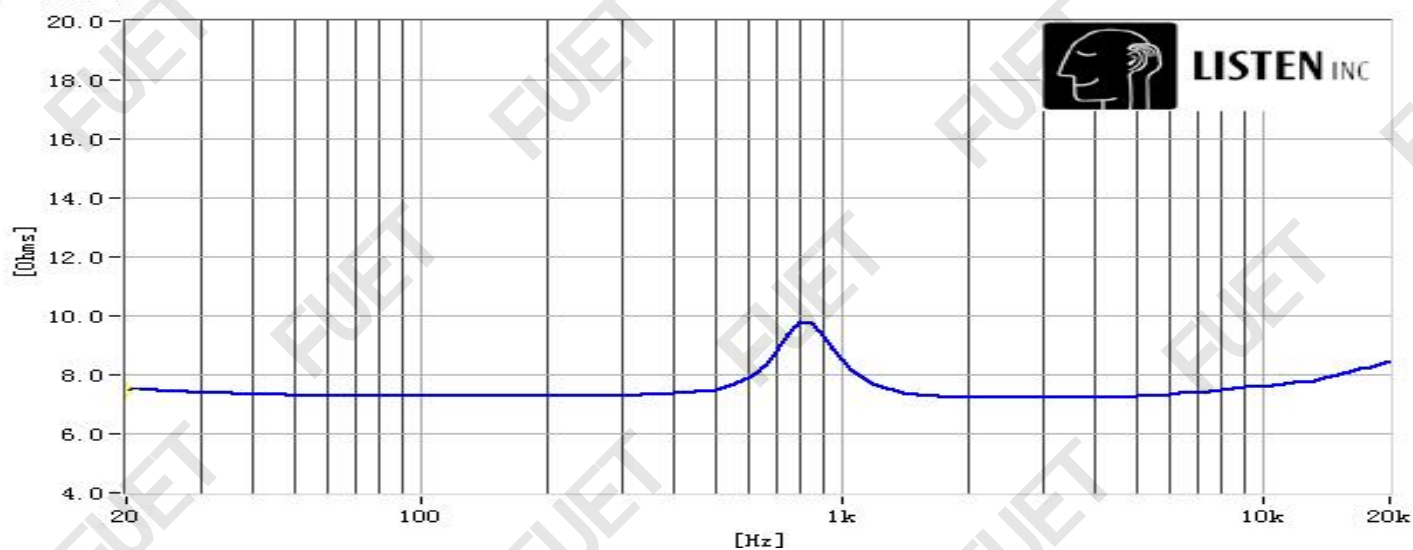
阻抗曲线
