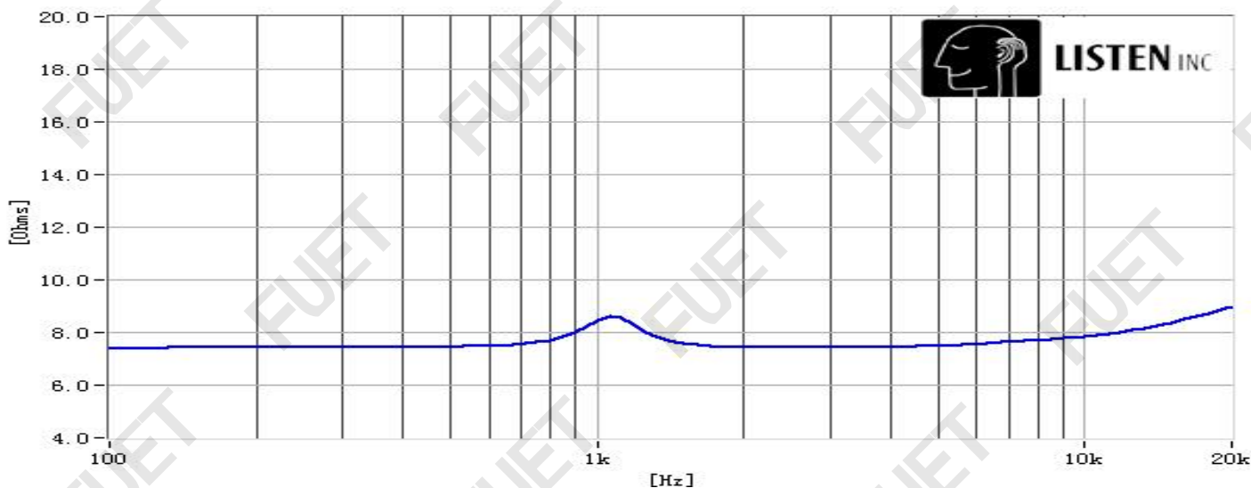
阻抗曲线
