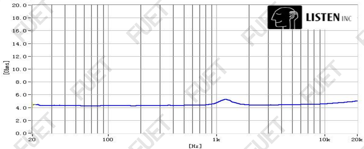
阻抗曲线
