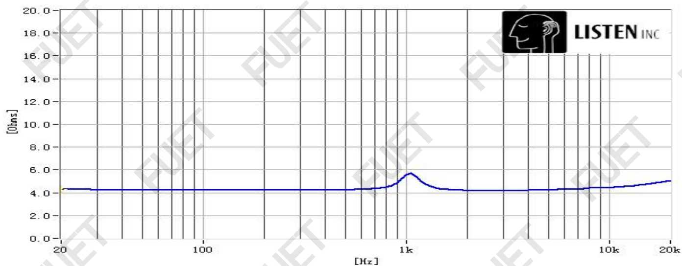
阻抗曲线
