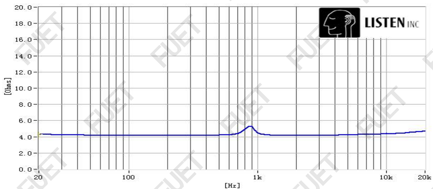
阻抗曲线
