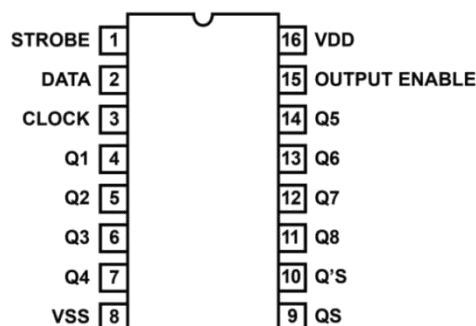
DIP-16/SOP-16/TSSOP-16
