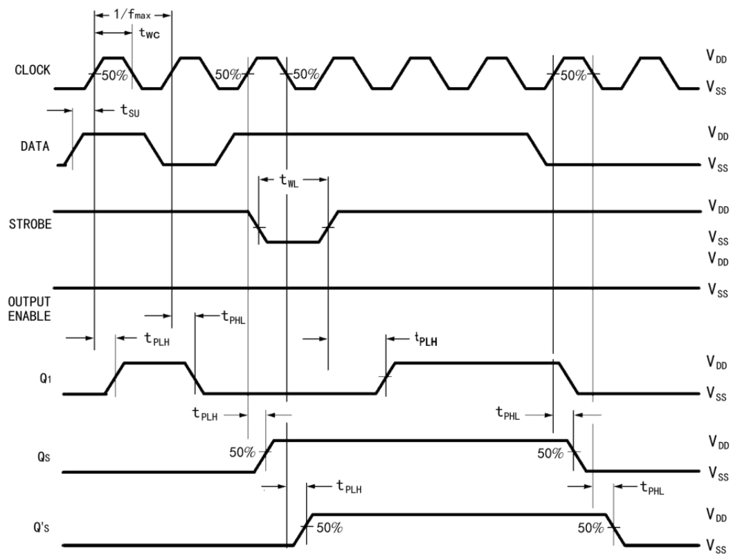
图 2: 时钟-输出传输延迟, 脉冲宽度, 最大频率
