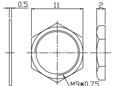
NUT 1pcs
