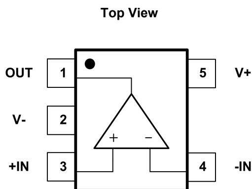
Fig.5-2. GT321B: S5(SOT23-5) Package
