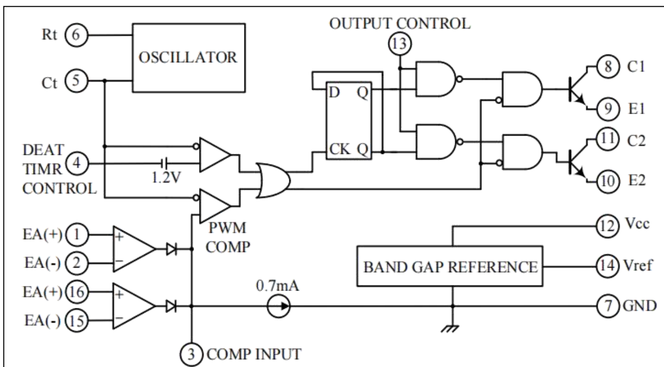
图 1 KA7500B 原理图
