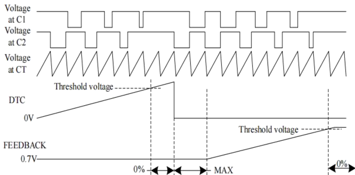
图 6 电压波形
