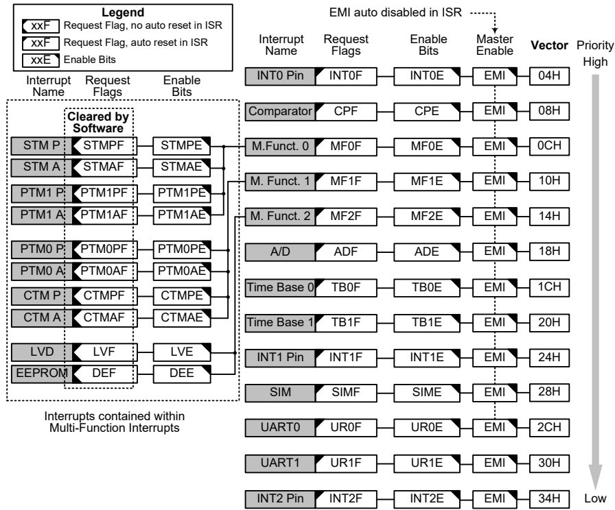
中断结构
