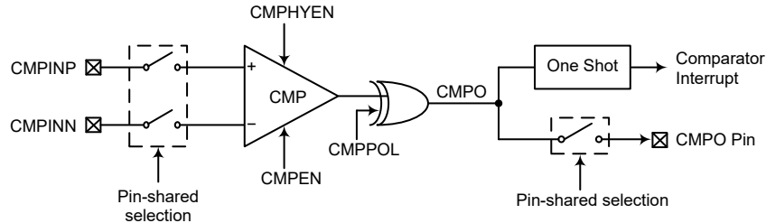
比较器
